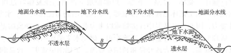
图 1-2 流域地面和地下分水线示意图
