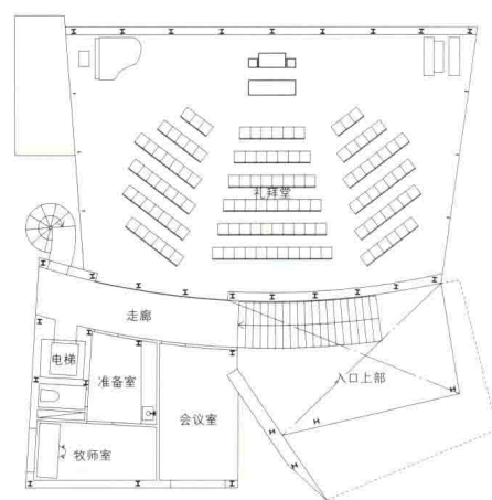
2层平面图
