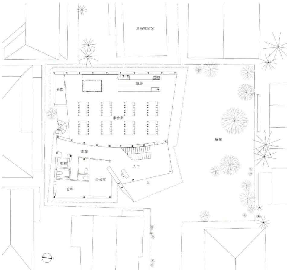
1层平面图 比例尺1:300
