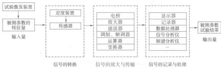
图 1-1 典型的试验测试系统的组成框图
