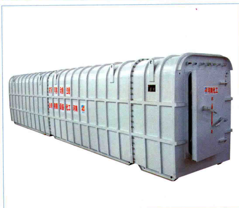
+ 矿用可移动分体式救生舱
