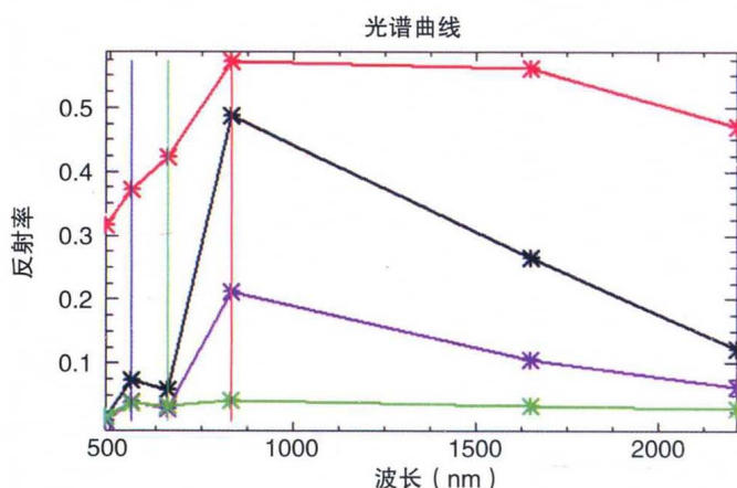
1995年影像中的端元选取和提取的端元光谱曲线
