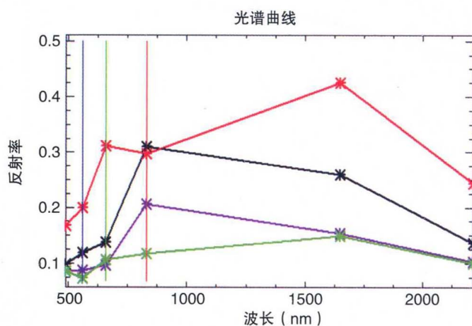
2000年影像中的端元选取和提取的端元光谱曲线
