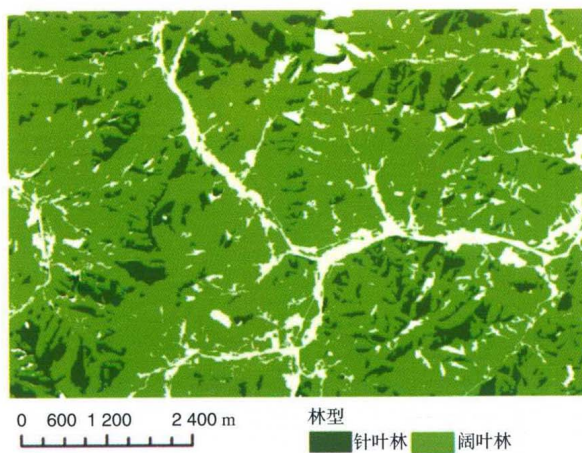
图6-23 面向对象分类结果图
