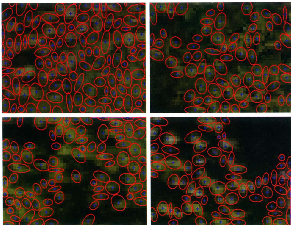
图6-44 部分样地树冠提取结果图
