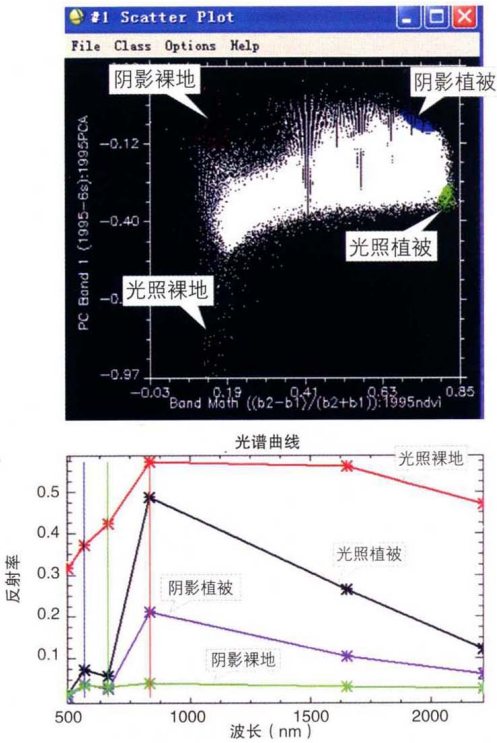
图5-5 基于PC1和NDVI的端元选取
