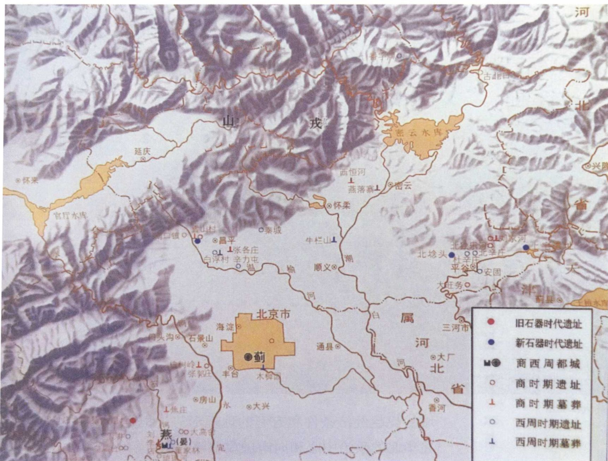
古代北京地区的地理形势
