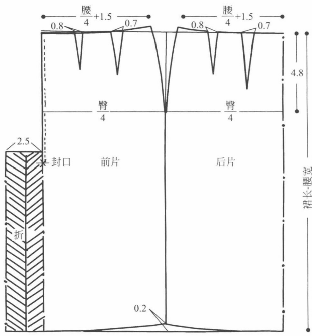
暗裱裙裁剪制图
