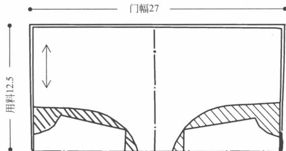
排料图之二（对折排料）
