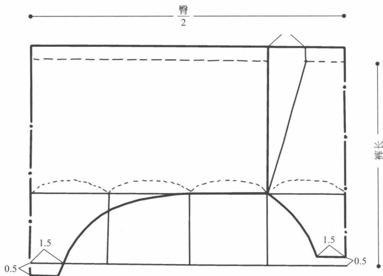
排料图之一（四折排料）
