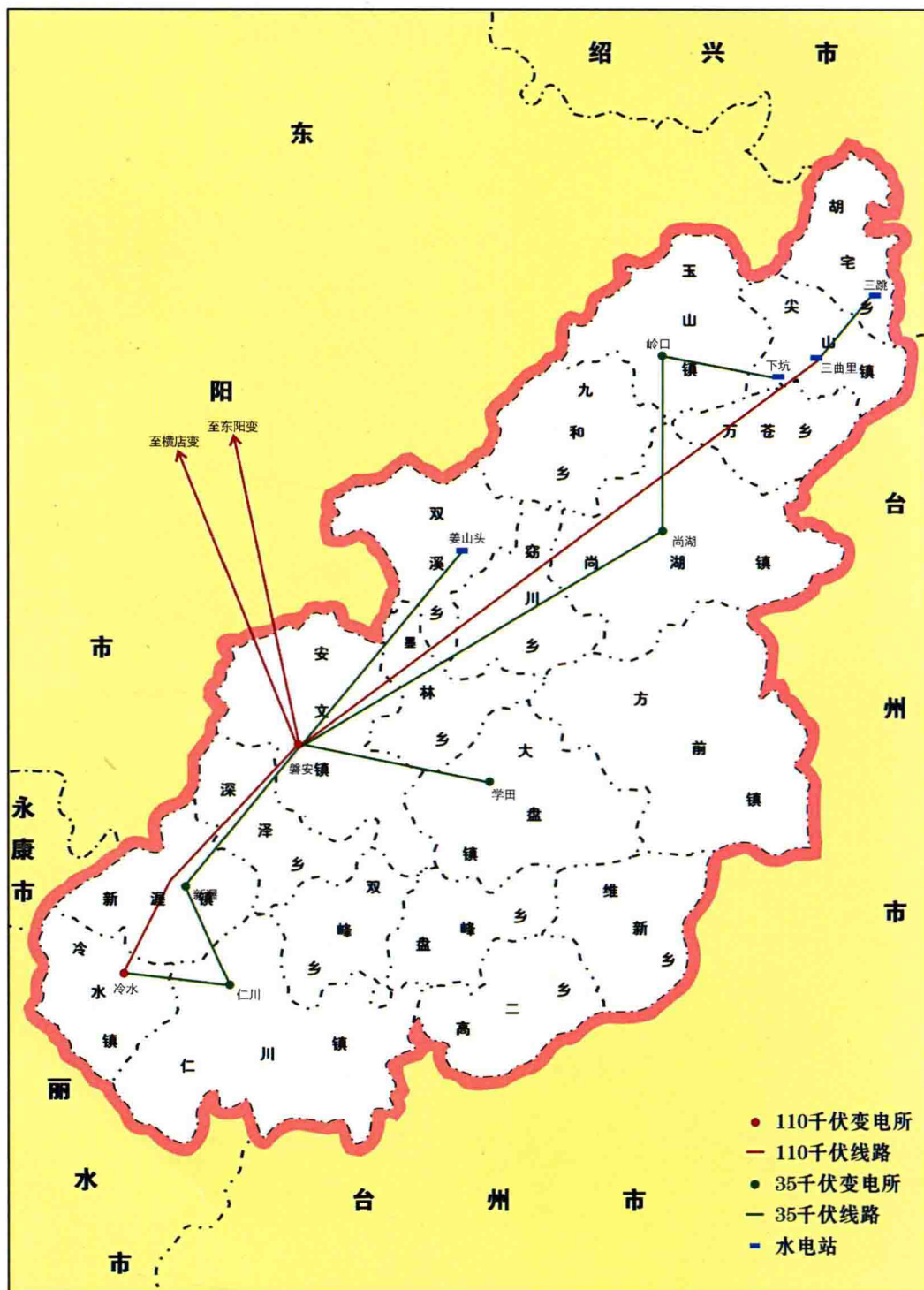
2005 年磐安县电网地理接线示意图
