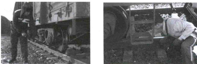
图 1-6 铁鞋制动
