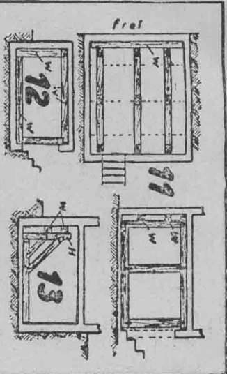
Sicherung der Schutzraum-Seitenwände.
