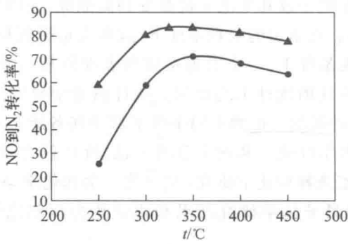
图 0.1 NO 到 N 2 的转化率与温度的关系 (● 在 HZSM-5 上 ▲ 在 3%Y/HZSM-5 上)
