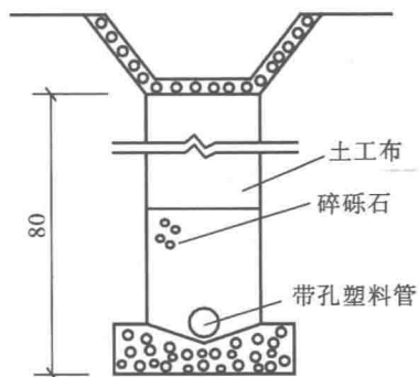
图 1-9 1号路盲沟构造示意图
