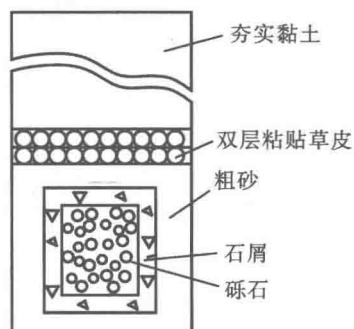
图 1-12 2 号路盲沟构造示意图
