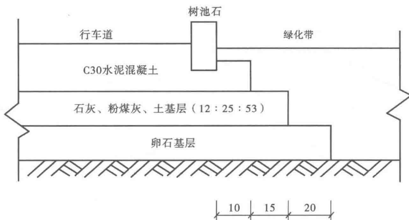
图 1-14 2 号路树池构造示意图
