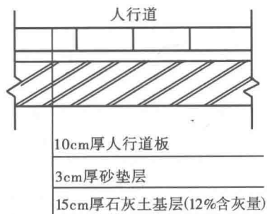
图 1-8 1号路人行道结构示意图
