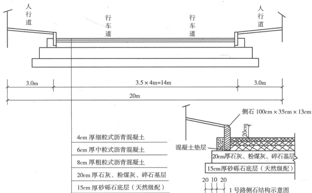
图 1-2 1 号路路面结构示意图
