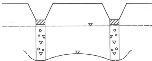
图 1-7 1号路路基纵向盲沟双列式示意图
