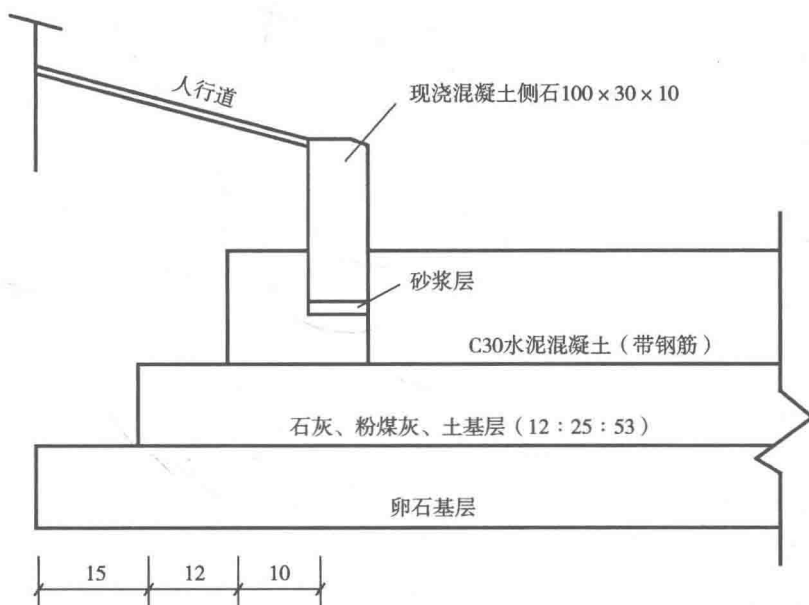
图 1-13 2 号路侧石构造示意图(单位:cm)
