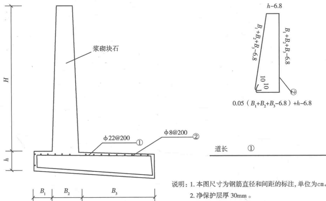
图 1-6 挡土墙配筋示意图
