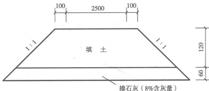
图 1-10 2号路路基断面示意图
