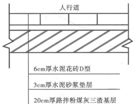
图 1-11 2 号路人行道结构示意图
