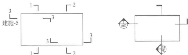
图 1.5 剖视的剖切符号
