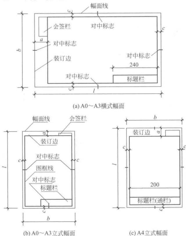
图 1.1 图框形式
