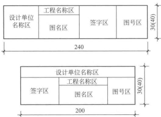
图 1.2 标题栏
