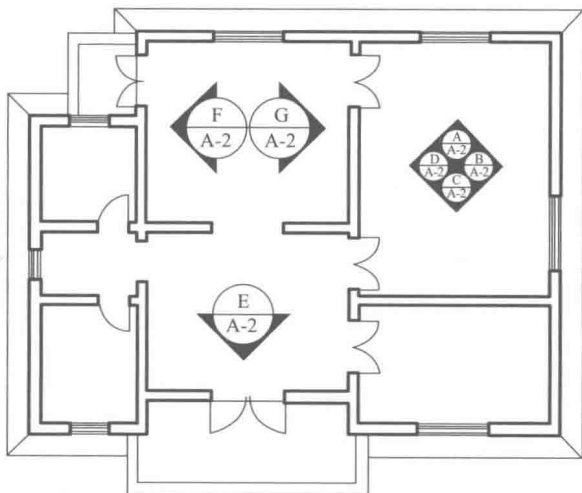
图 1.10 平面图上内视符号（带索引）应用示例
