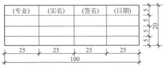
图 1.3 会签栏
