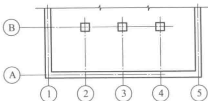
图 1.15 定位轴线示意 (平面图局部)
