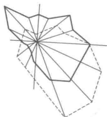
图 1.13 风玫瑰图
