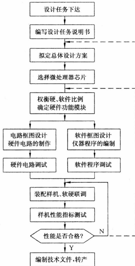
图 1-5 设计、研制智能仪器的一般过程
