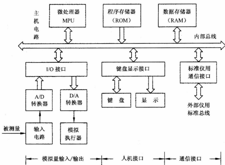
图 1-1 智能仪器基本结构框图
