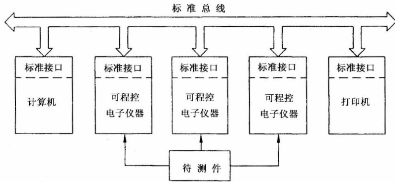
图 1-2 典型自动测试系统
