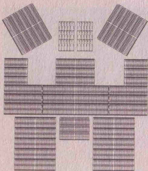
◎ 明代铁甲复原展开示意图
