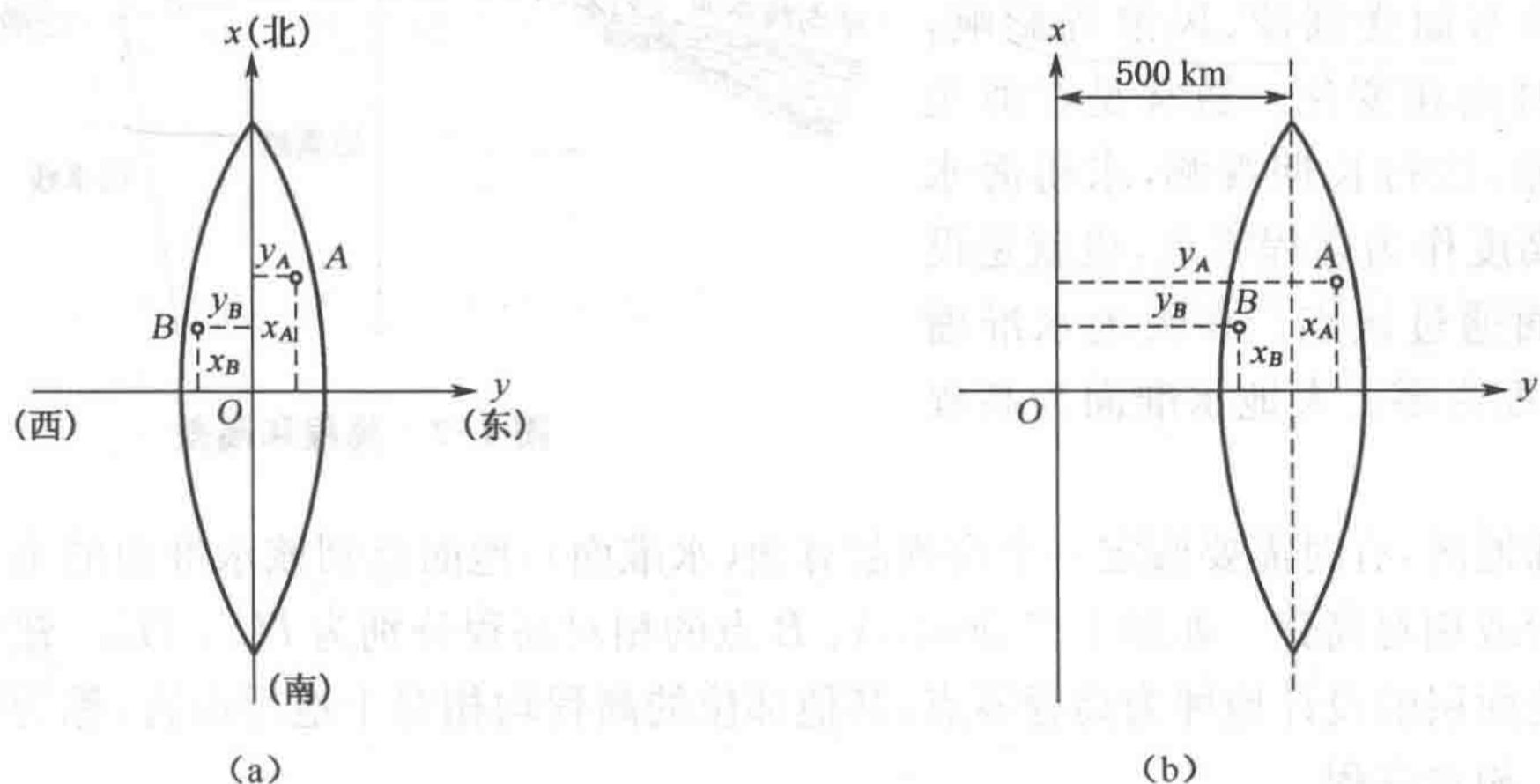
图 1-6 高斯平面直角坐标
