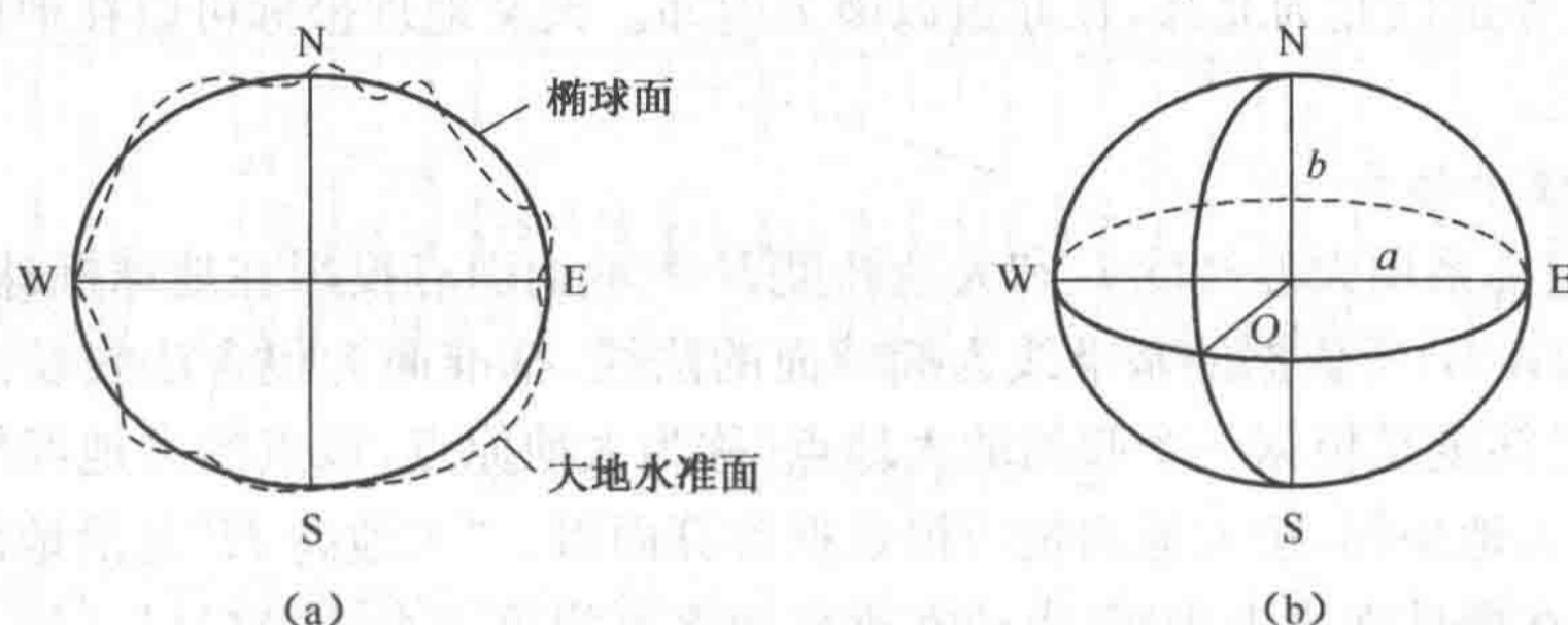
图 1-1 大地水准面与地球椭球体
