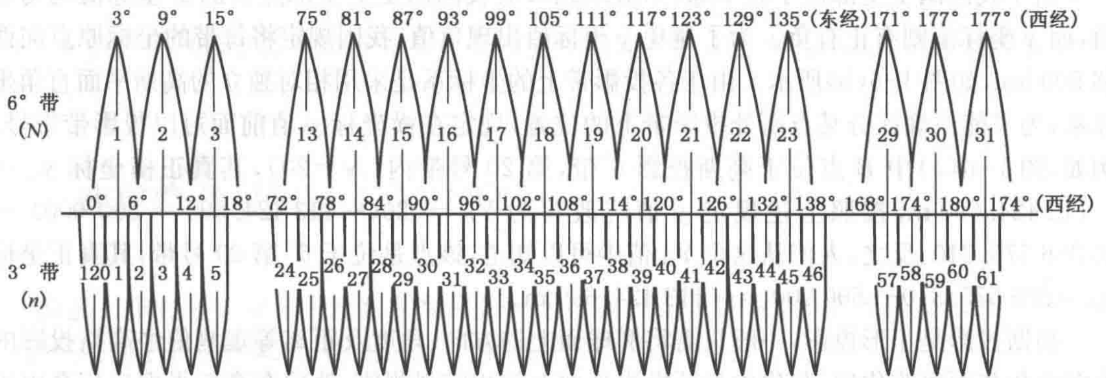
图 1-4 投影分带与 6°(3°)带
