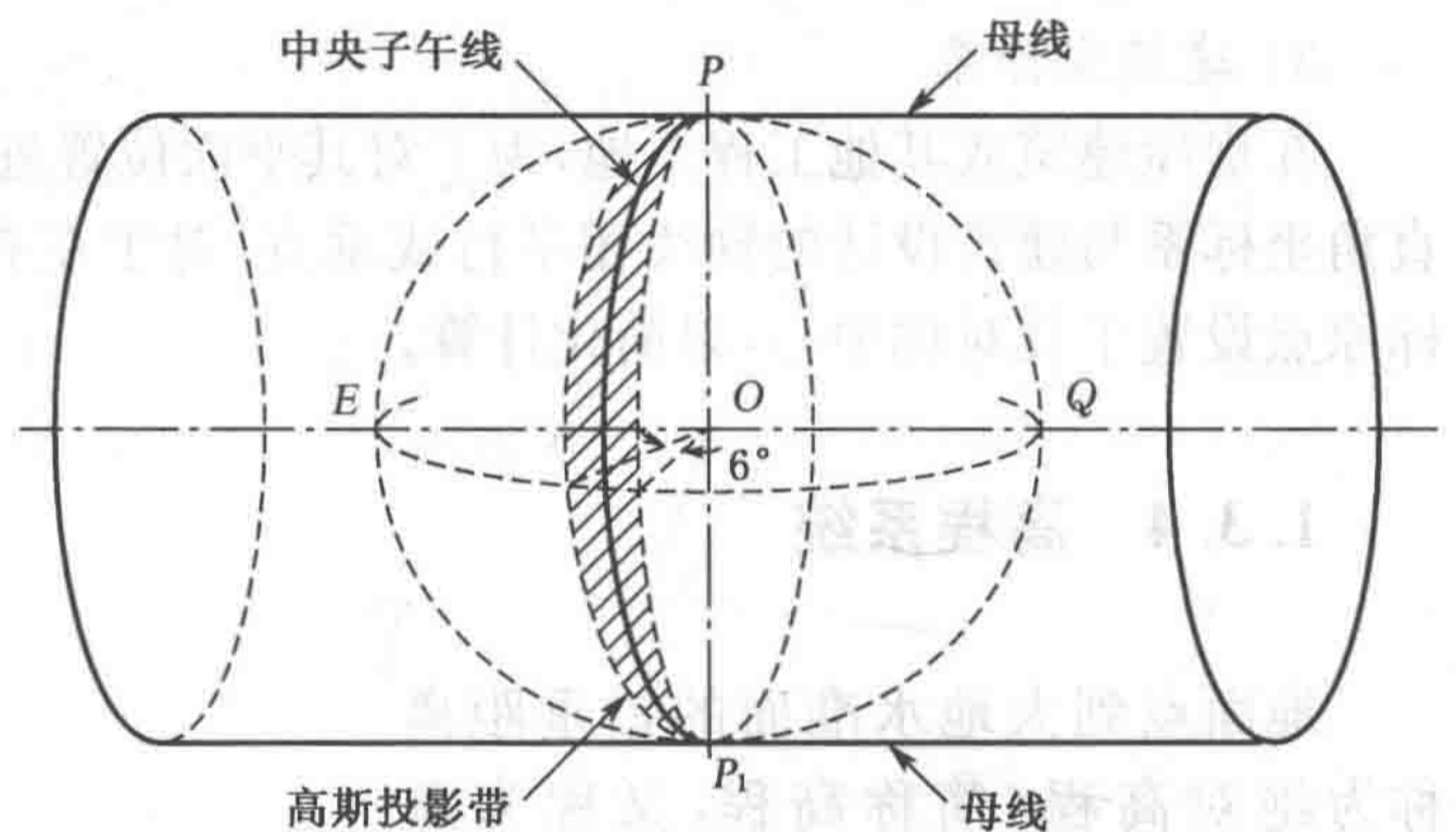
图 1-5 高斯平面直角坐标的投影
