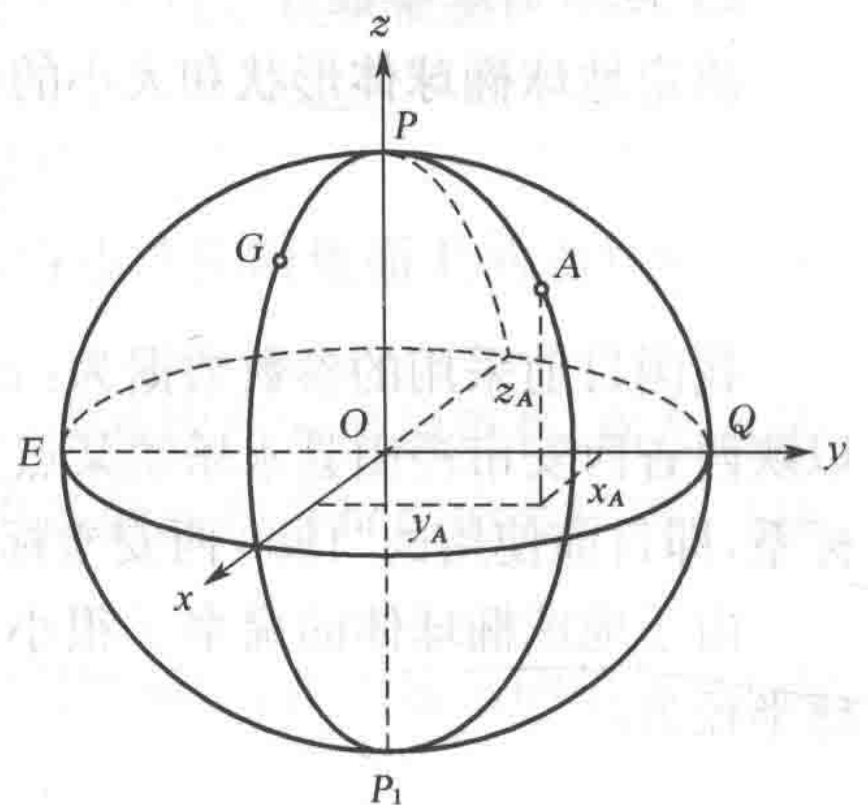
图 1-3 地心坐标系
