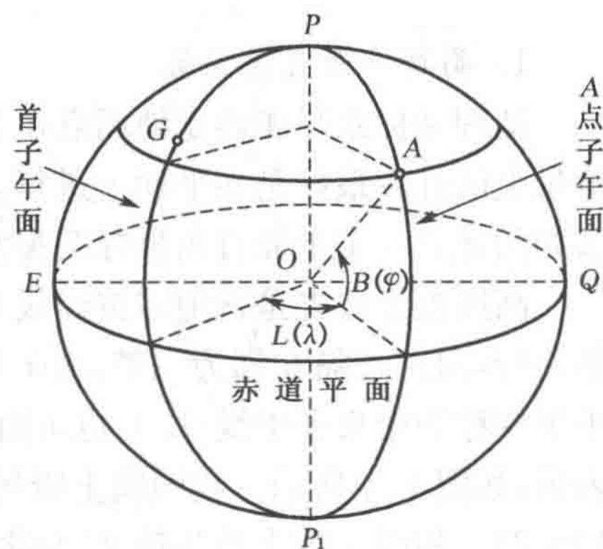
图 1-2 大地地理坐标系
