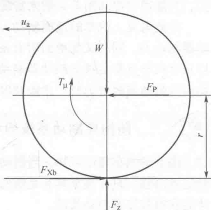
图 1-4 车轮在制动时的受力分析
