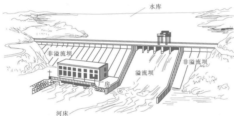
图 0.4 坝后式水电站
