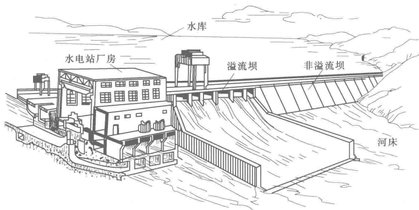
图 0.3 河床式水电站
