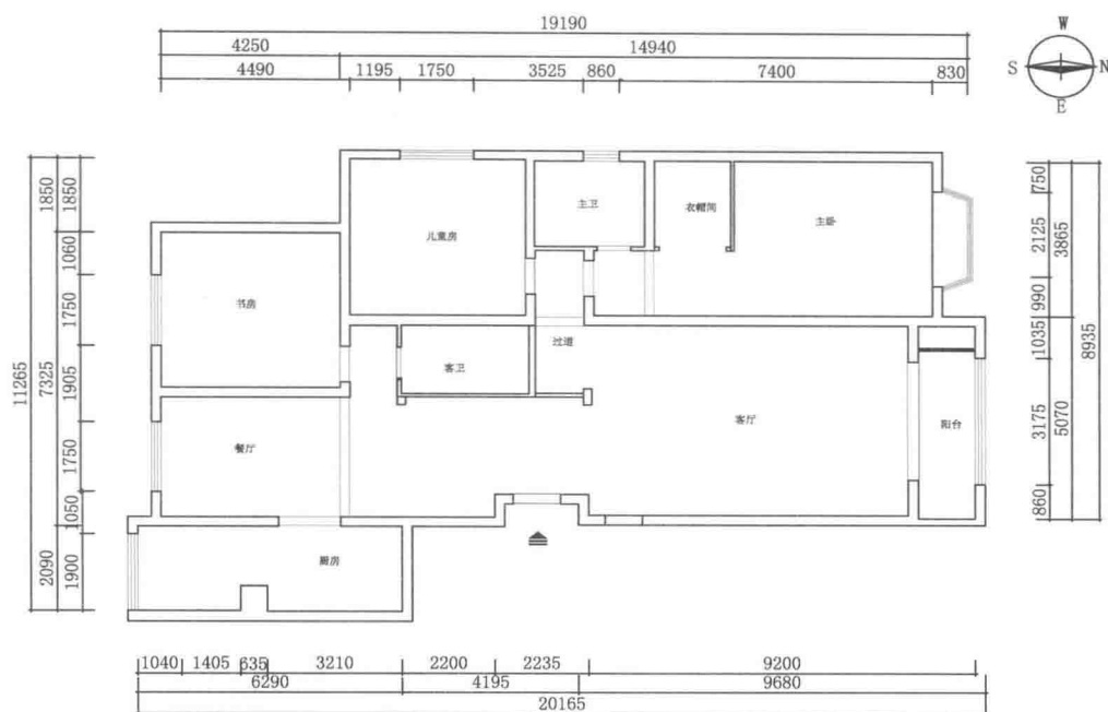
改造后平面布置图 1:80
