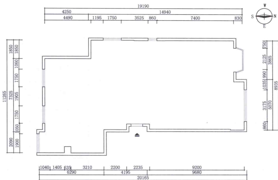
图 2-4-2 原始结构图
