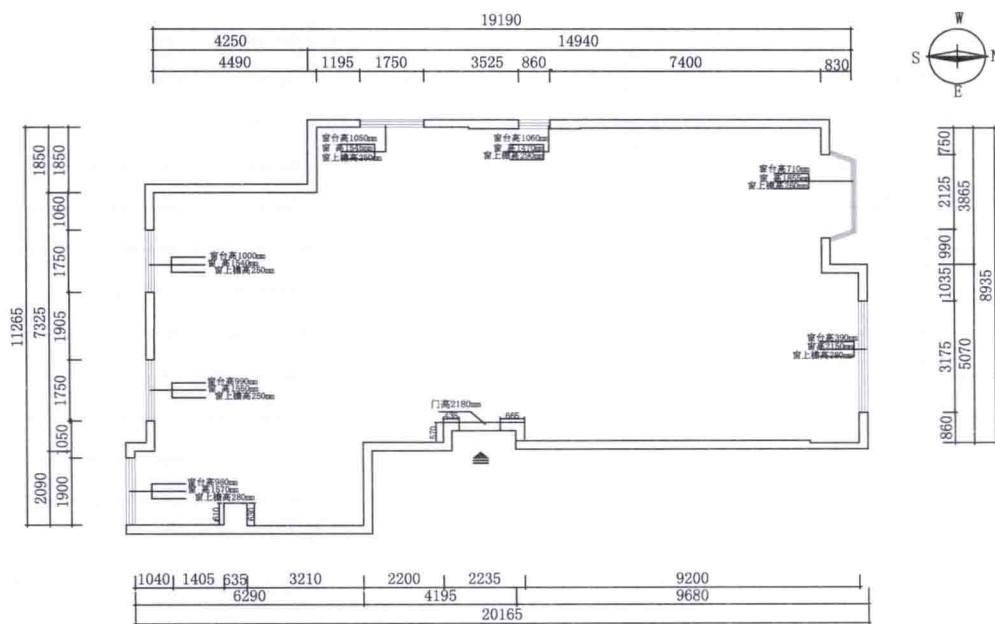
图 2-4-3 原始量房尺寸图
