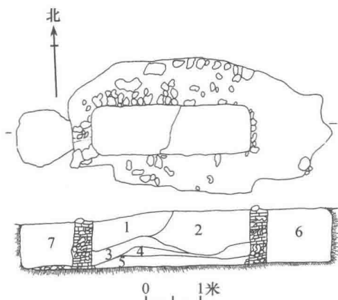
图3.4-3 东坪遗址1988年13号炼炉平、剖面图
