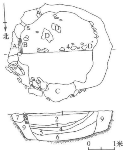
图3.4-4 东坪遗址1988年5号炼炉平、剖面图
