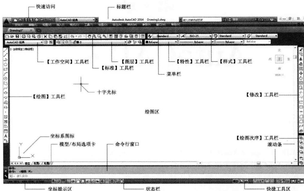
图 1-2 【AutoCAD 经典】工作界面
