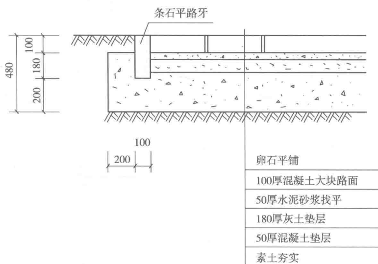
图 1-4 条石平路牙及路面详图
