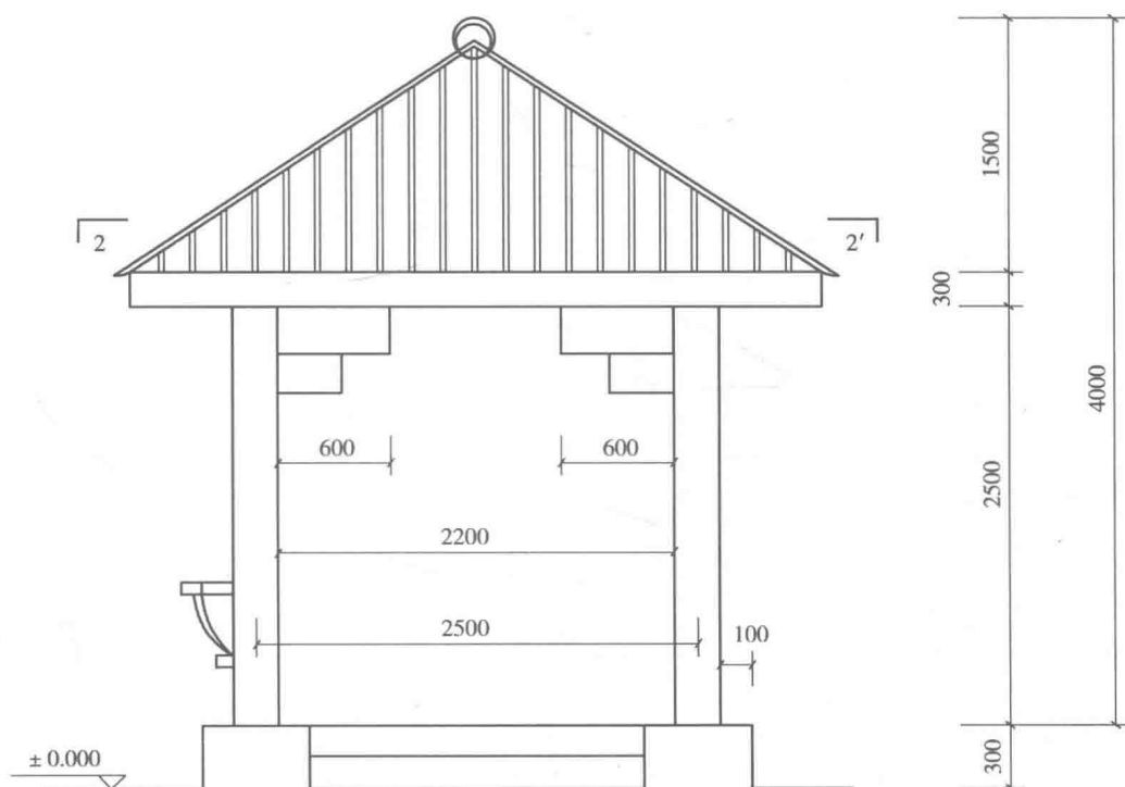
图 1-20 亭子正立面图
