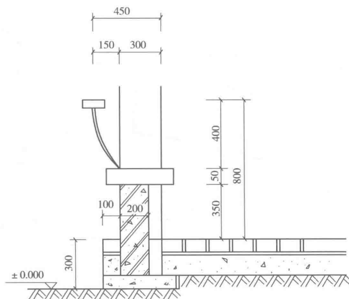
图 1-21 座椅剖面图
