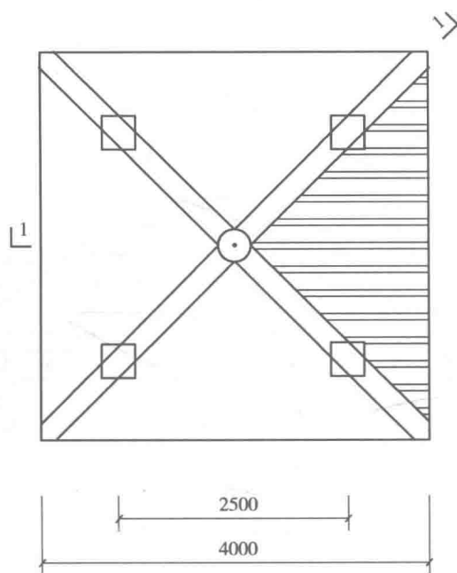
图 1-19 屋顶平面图
