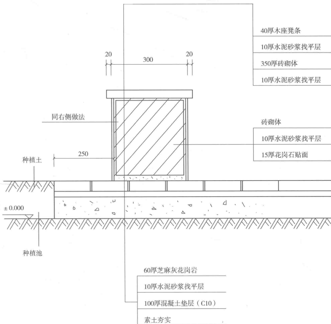
图 1-13 座凳剖面大样
