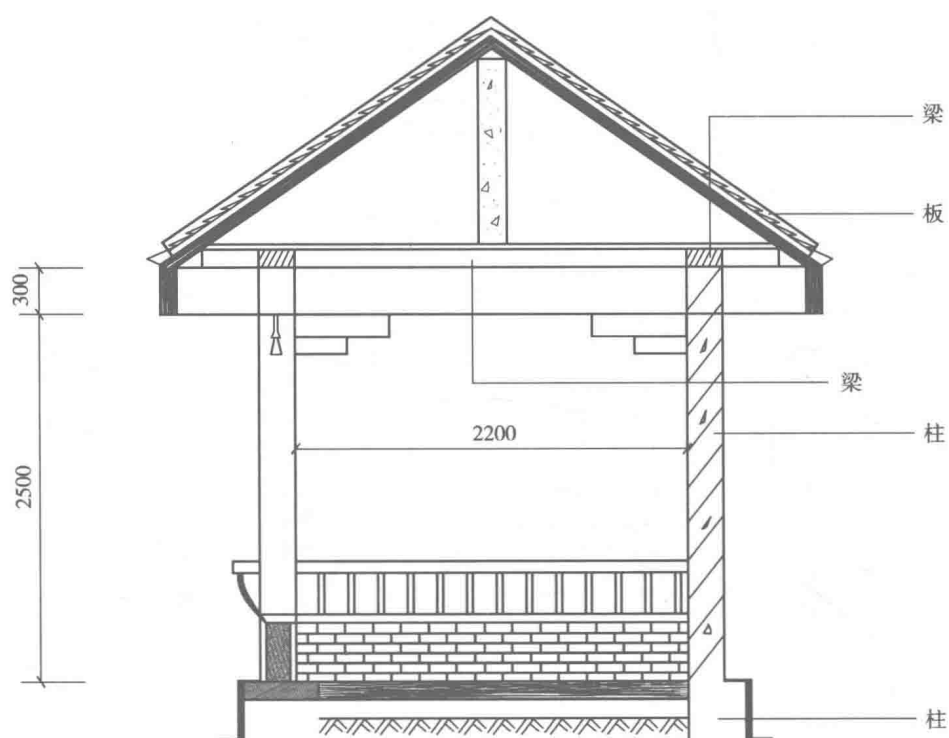
图 1-18 屋顶剖面图
