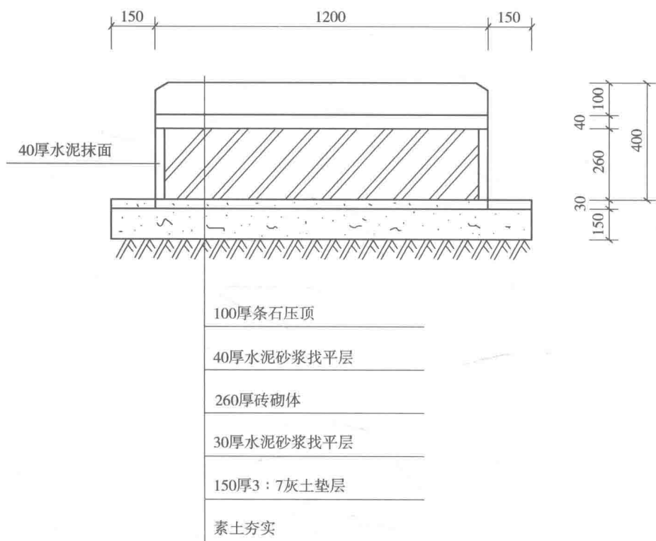
图 1-11 座凳剖面图
