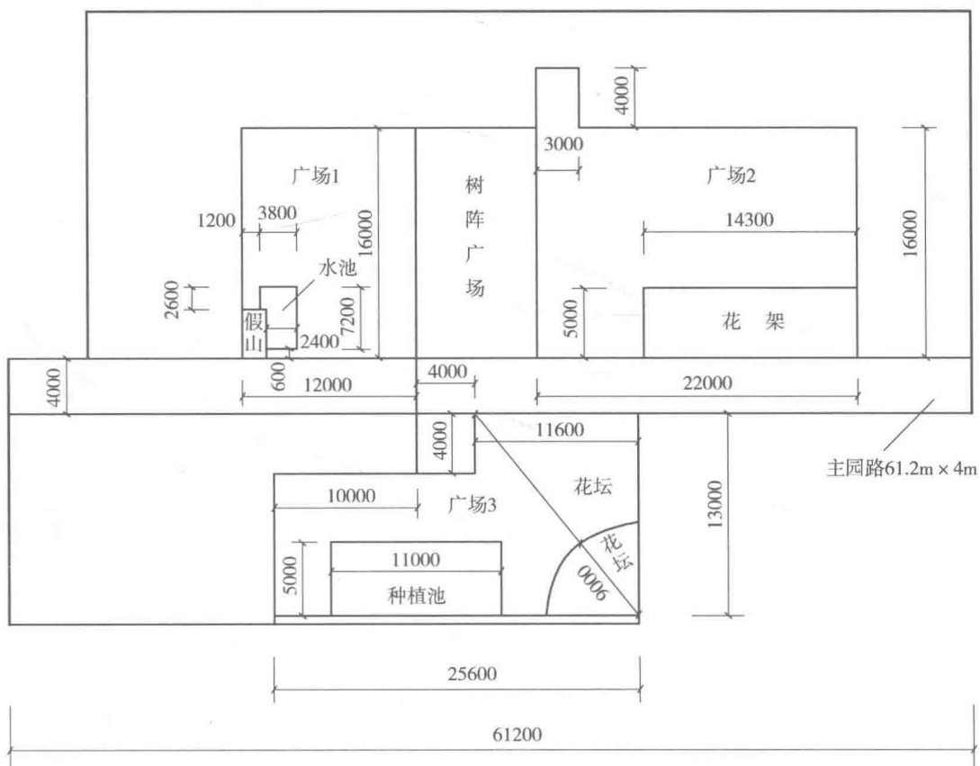
图 1-8 平面尺寸详图
