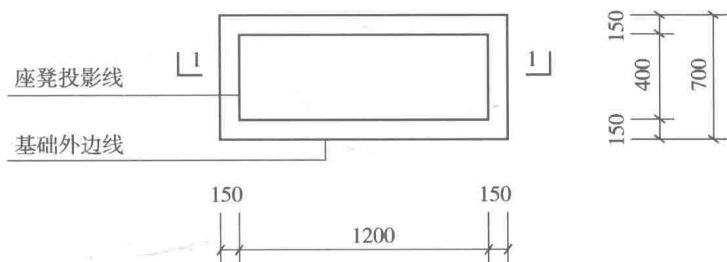
图 1-12 座凳基础平面图
