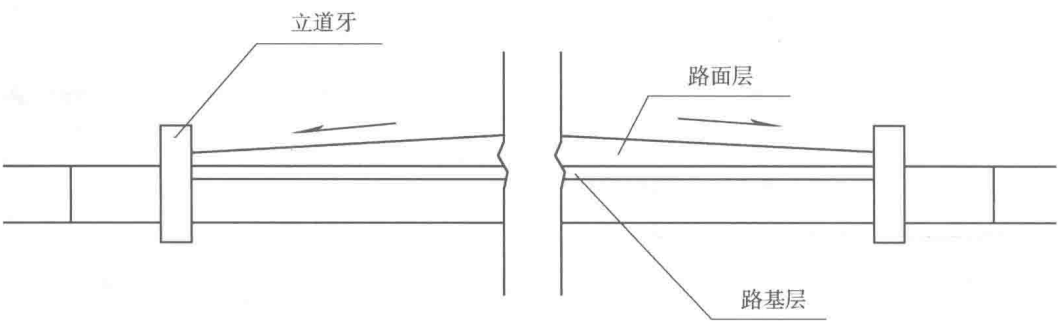
图 1-5 立道牙示意图
