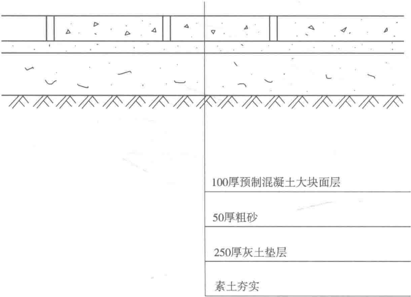
图 1-7 广场剖面示意图
