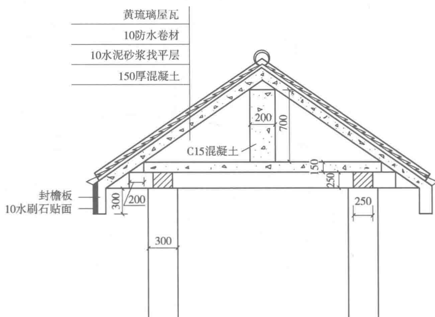
图 1-17 屋顶剖面详图
