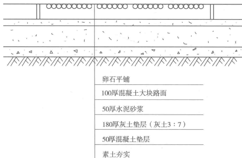
图 1-3 园路剖面图
