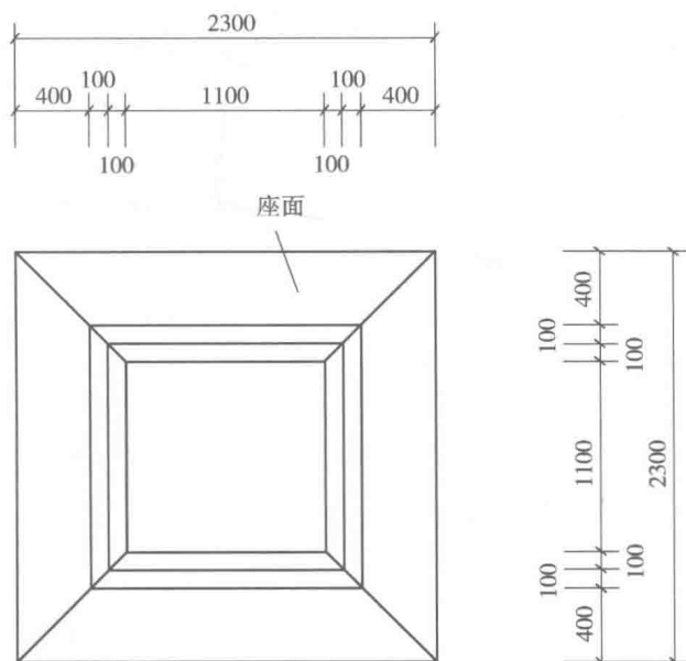
图 1-9 围树椅平面图
