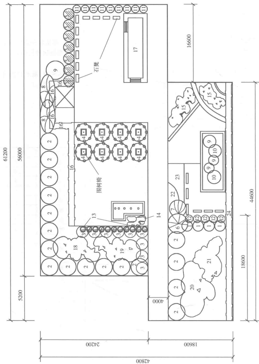
图1-1 总平面图
