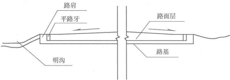
图 1-6 平路牙示意图
