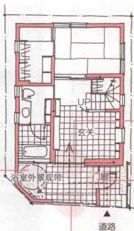
初台的住宅 1F 1:200
