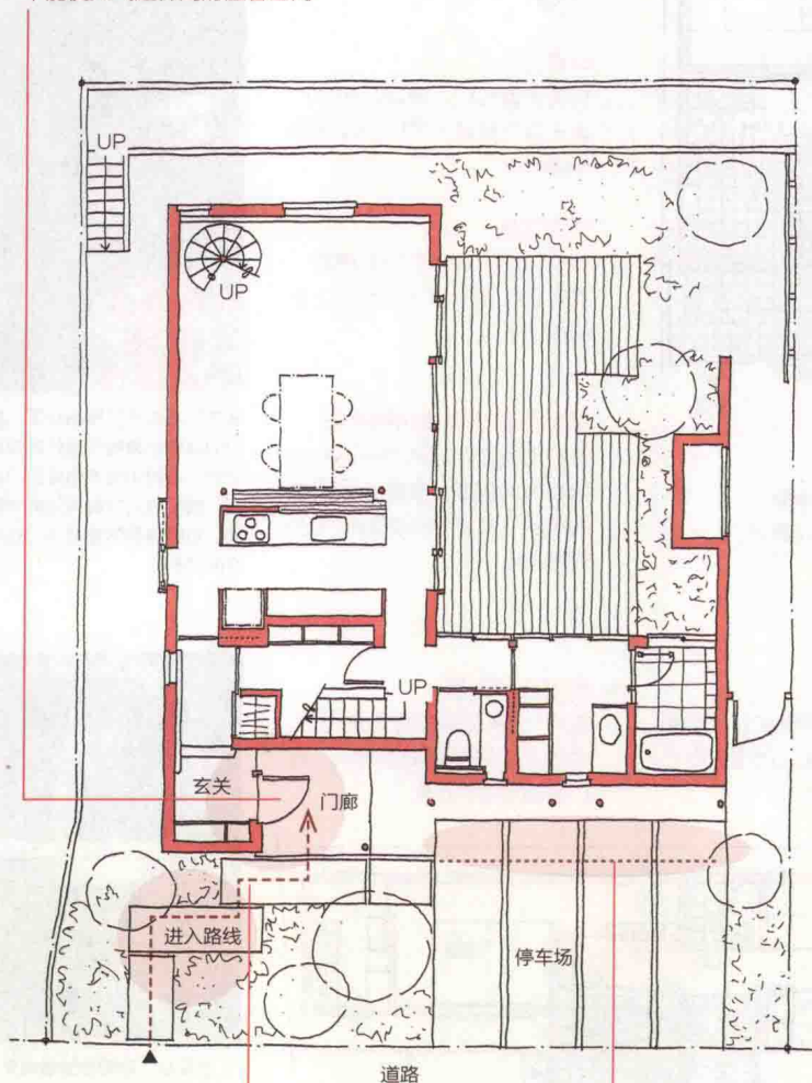
鸠山的住宅 1F 1:150
