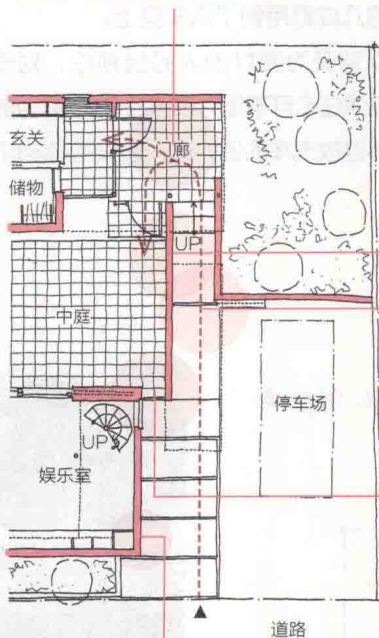
田园调布的住宅 1F 1:200
