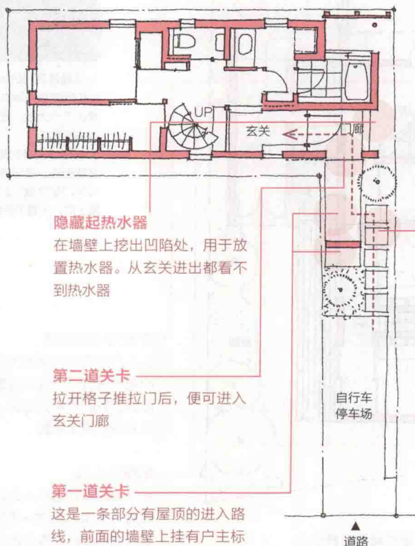
下高井户的住宅 1F 1:150
