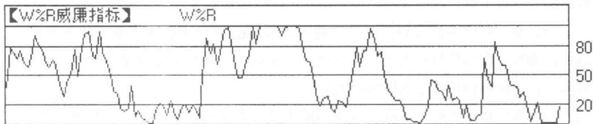
图1-1 威廉指标示意图
