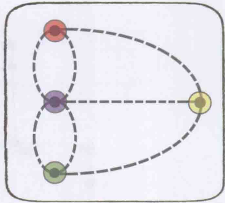
图 4-30 柯尼斯堡七桥问题简化图
