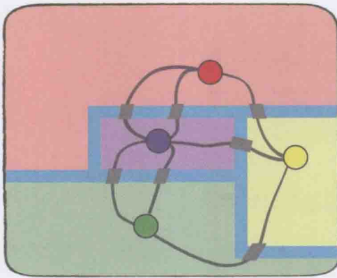
图 4-29 柯尼斯堡七桥问题原理图
