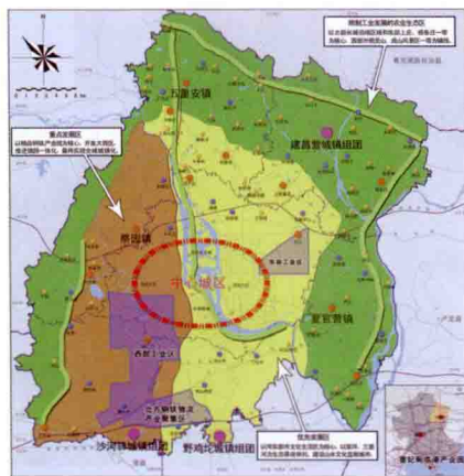
三大主体功能区划图
